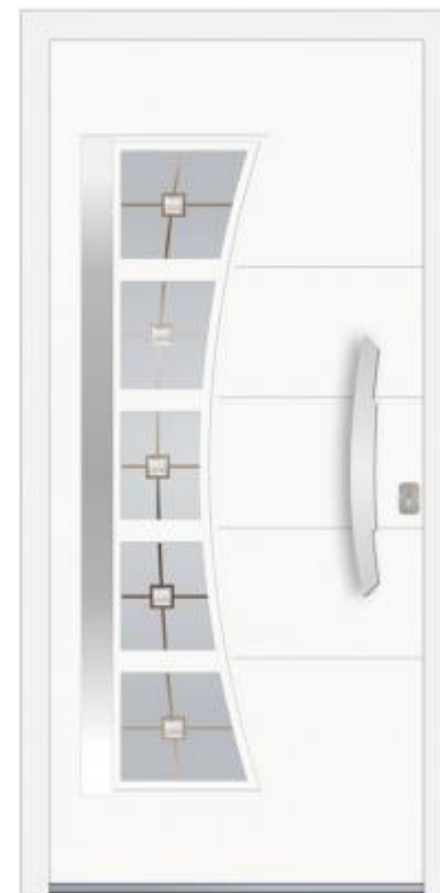
Farbe: 9016 glanz Glas: PFB Applikation: INOX zweiseitig Handgriffe: GPS 115h Rosette: RKM 30
